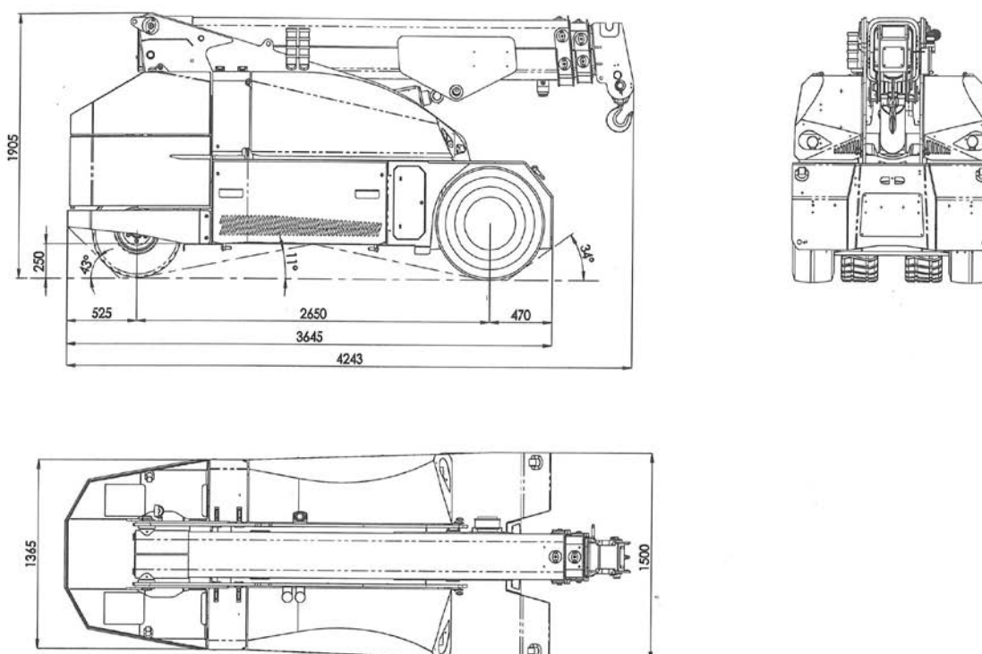
Fig. VII. Viste standard della gru
